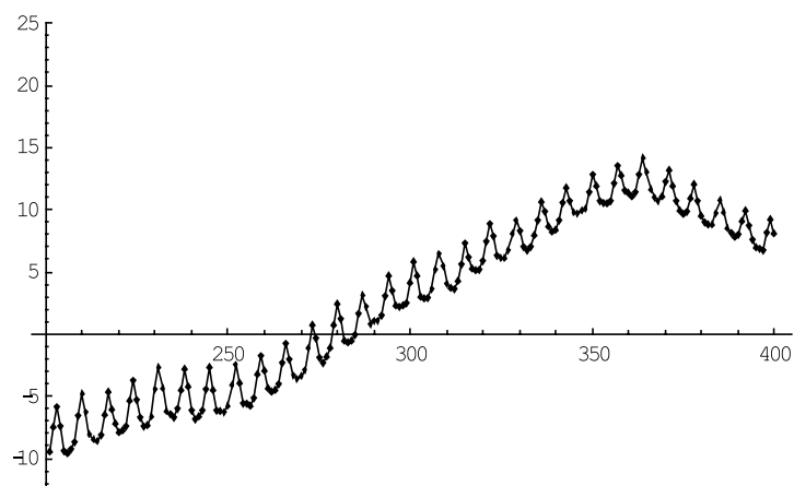
Rysunek 4. Wykres funkcji korelacyjnej K(\tau) dla \tau \in \langle 201, 400 \rangle
