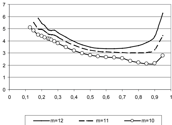
Rysunek 7. Wykresy funkcji d_C(r, \tau^*) = \frac{\log C(r, \tau^*)}{\log r} dla \tau^* = 2 dla wybranych poziomów m
