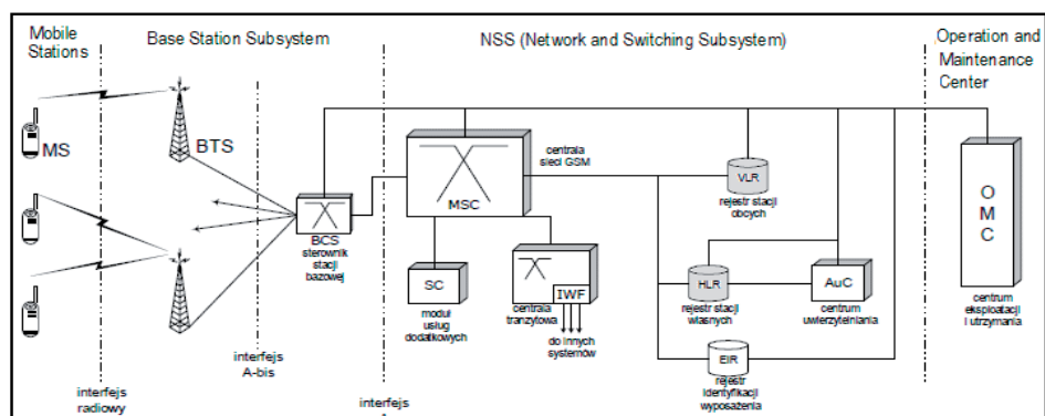
Rysunek 1. Architektura systemu GSM
