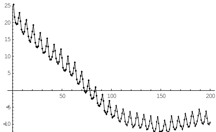
Rysunek 3. Wykres funkcji korelacyjnej K(\tau) dla \tau \in \langle 1, 200 \rangle
