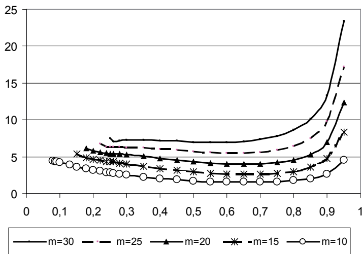
Rysunek 6. Wykresy funkcji d_C(r) = \frac{\log C(r)}{\log r} dla wybranych poziomów m
