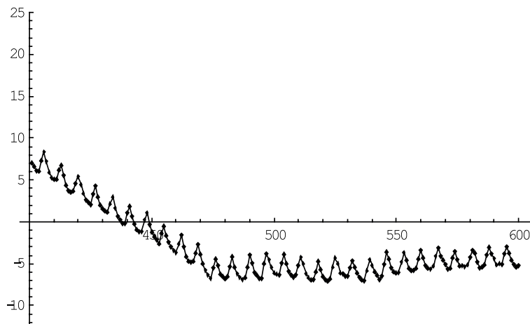
Rysunek 5. Wykres funkcji korelacyjnej K(\tau) dla \tau \in < 401, 600 >
